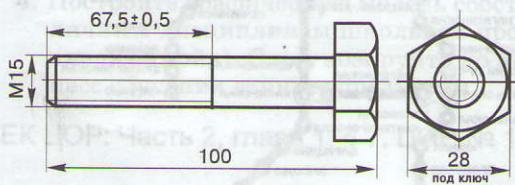
Рис. 2.3. Чертеж болта
