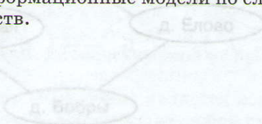
Рис. 2.9. Граф, отражающий связь между населенными пунктами
