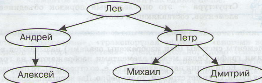
Рис. 2.11. Ориентированный граф родственных связей
