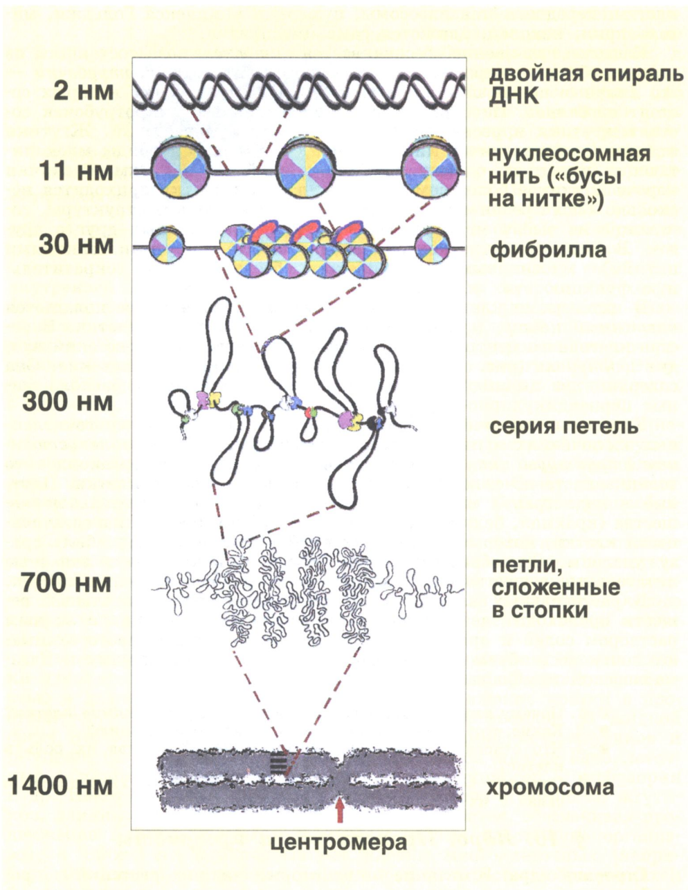
Рис. 17. Схема упаковки ДНК в хромосоме
