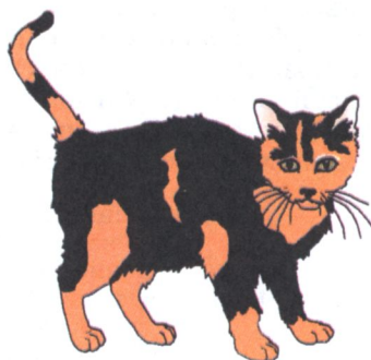
Рис. 41. Черепаховая окраска кошки
