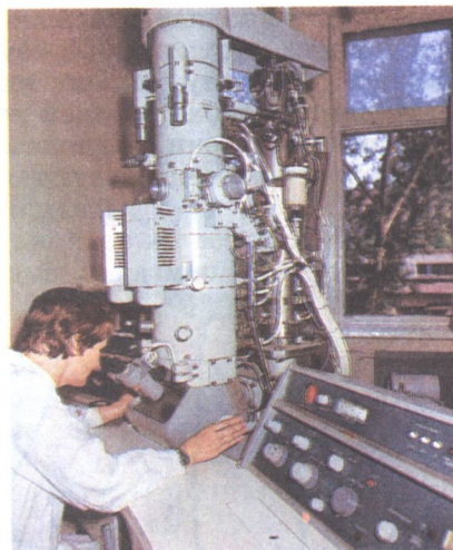
Рис. 9. Электронный микроскоп
