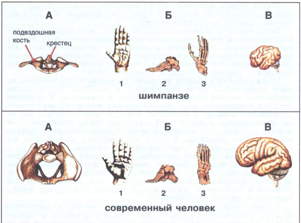
Рис. 90. Отличия в строении тела человека и шимпанзе.
